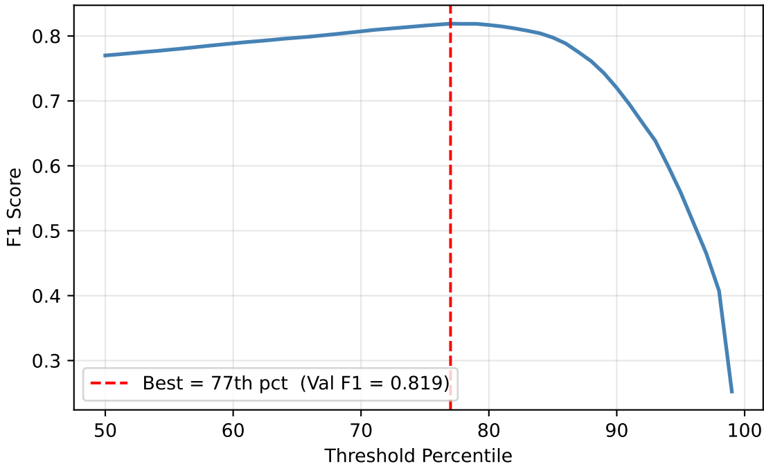
F1 vs Threshold Percentile
