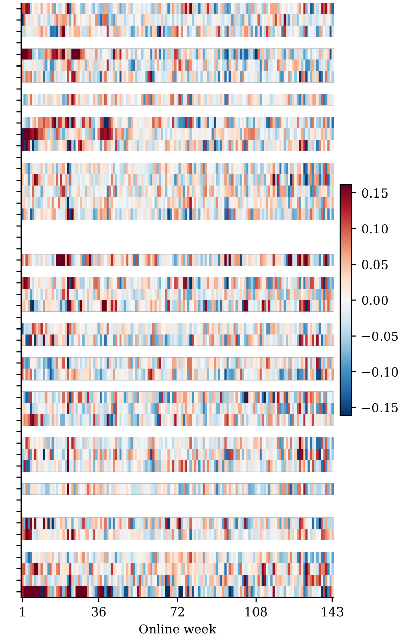
Ordinary - HiPPO error
