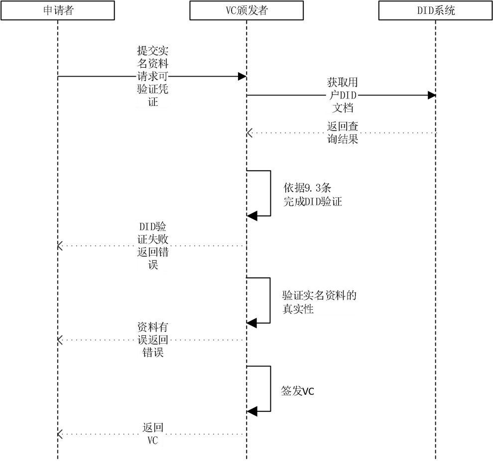
图 11 VC 颁发流程
