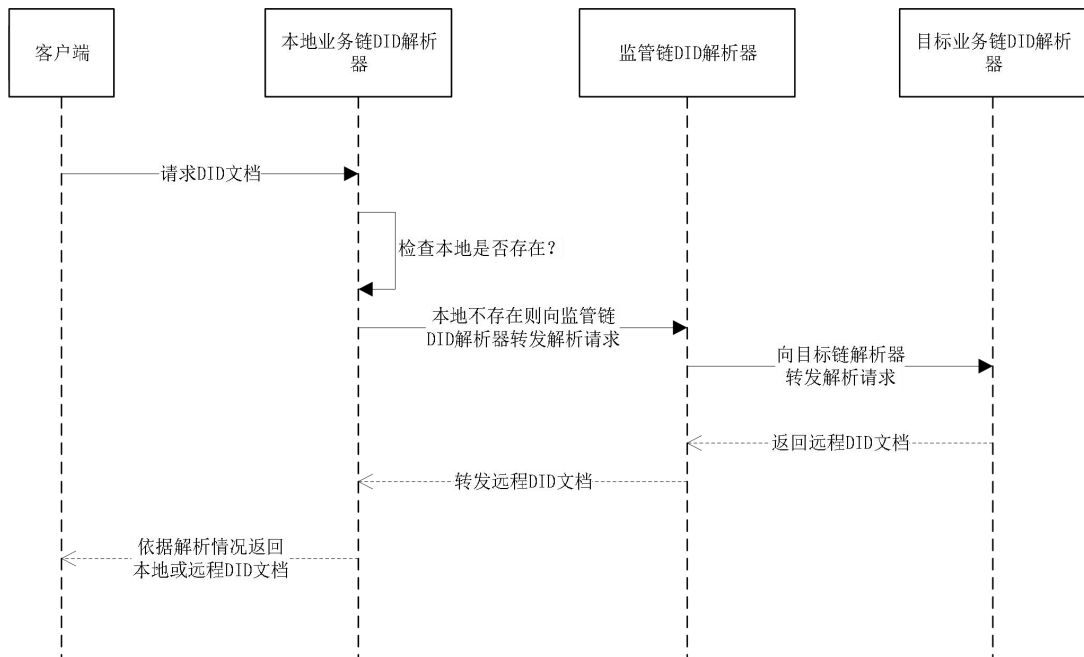
图 4 DID 解析流程
