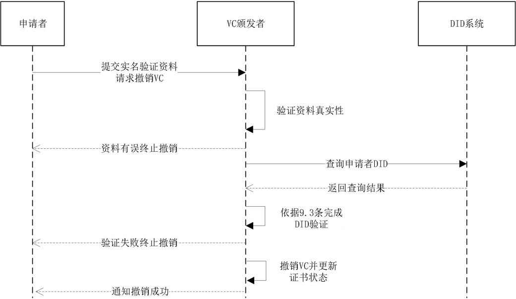
图 14 VC 撤销流程
