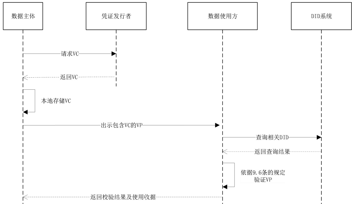
图 15 以数据主体为中心的数据流通流程
