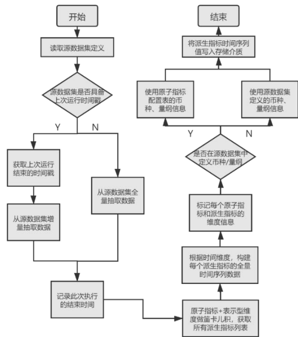
图 4 ETL 作业流程示意图
