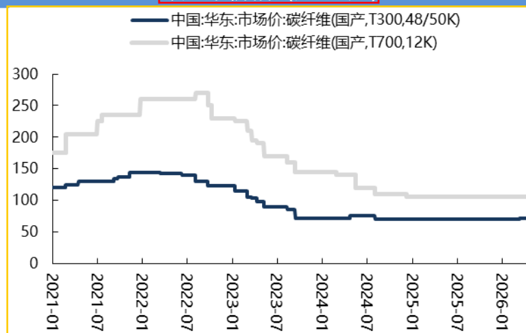
碳纤维价格 (元/千克)
