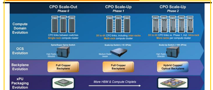
图 27：光通信技术演进拓展算力边界
