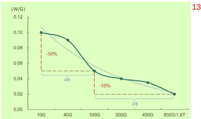
图表20：“光摩尔定律”下速率迭代与功耗演进趋势；光模块速率从400G向800G、1.6T演进
