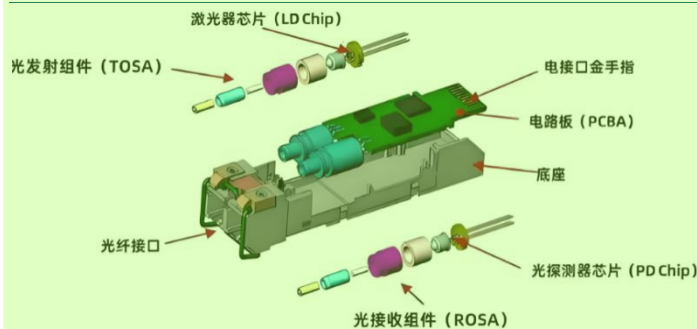
图表3：光模块包括光发射、接收及其他电路组件 11
