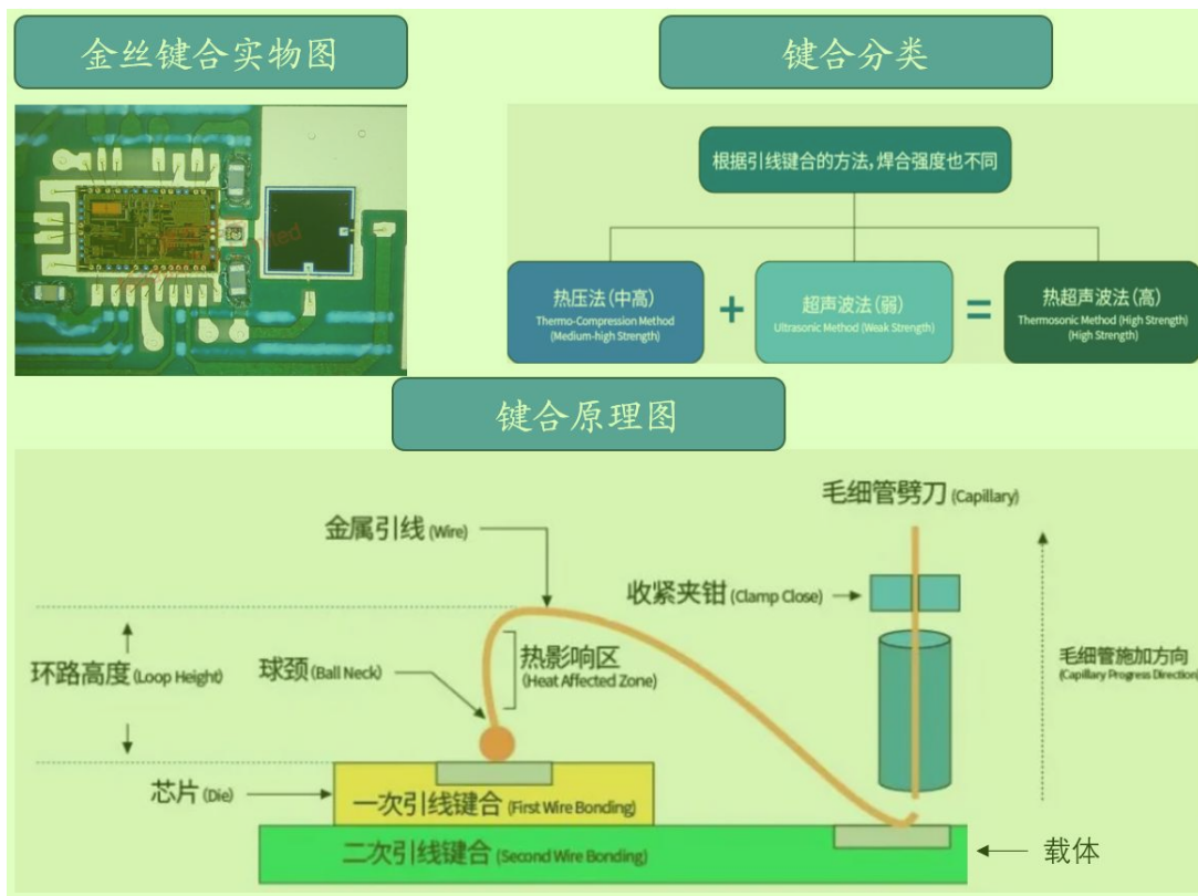
图表11: 光模块使用金丝球焊实现芯片引脚互联 6
