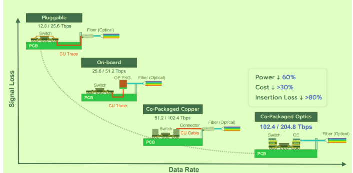
图表23：CPO 方案可降低 60% 的功耗和 30% 以上的成本 6
