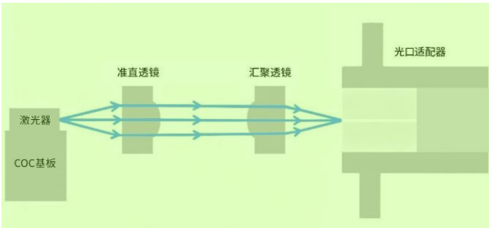
图表12：耦合在于将光芯片发射的光信号耦合进光纤 3
