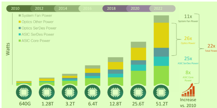
图表22：交换机带宽扩容带来核心部件功耗提升 3
