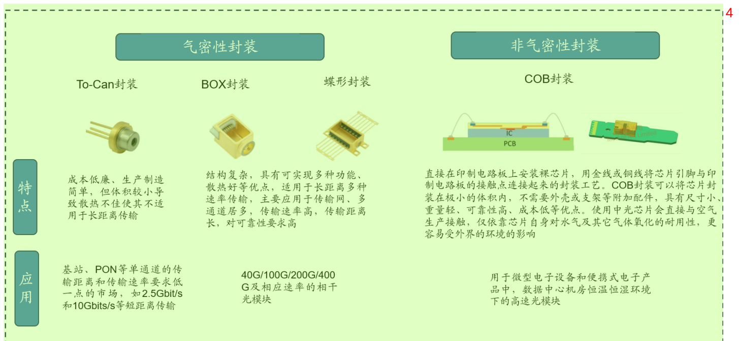
图表15：非气密性封装是高速光模块于数据中心机房应用的主流选择 3
