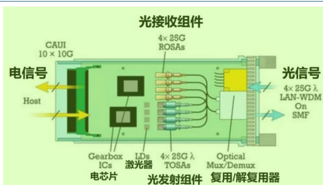
图表4：光模块通过其核心组件实现光电信号转换 13
