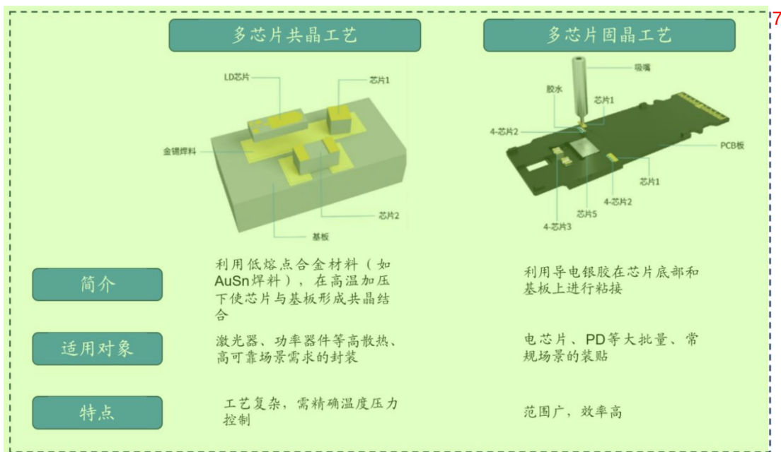
图表9：光模块贴装分为共晶和固晶两种工艺路线 6
