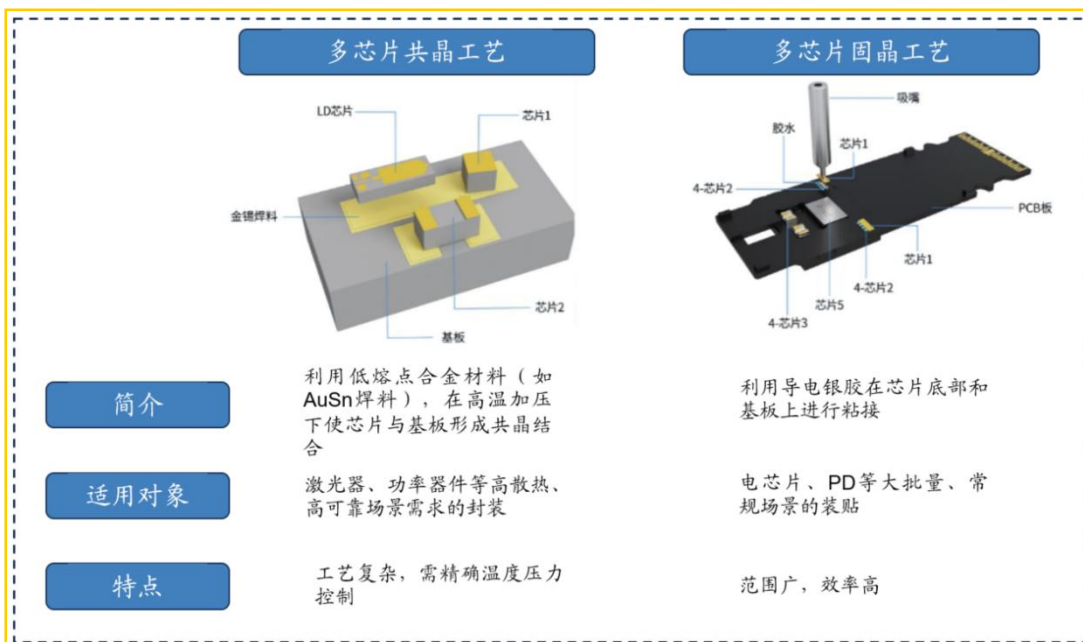
图表9：光模块贴装分为共晶和固晶两种工艺路线
