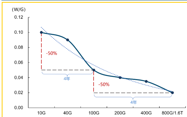
图表20：“光摩尔定律”下速率迭代与功耗演进趋势
