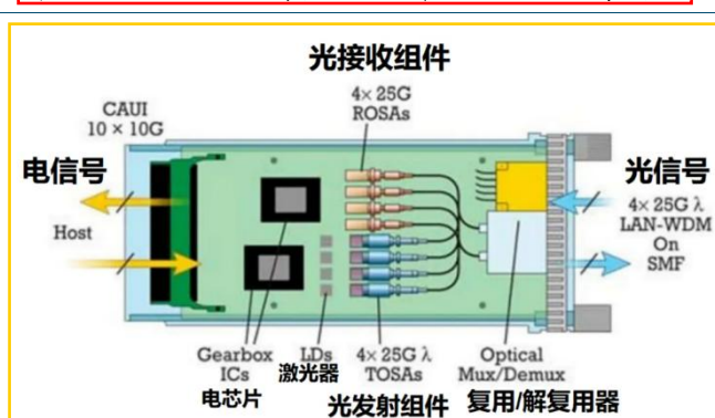
图表4：光模块通过其核心组件实现光电信号转换
