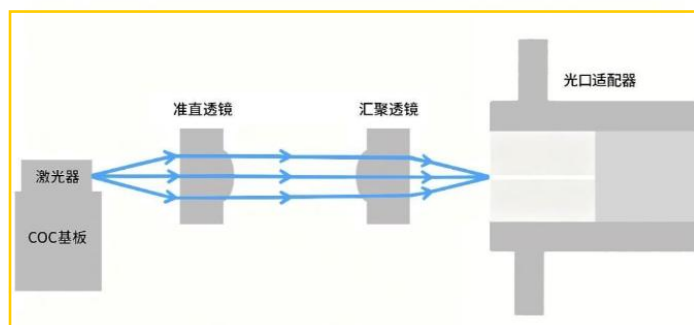
图表12：耦合在于将光芯片发射的光信号耦合进光纤
