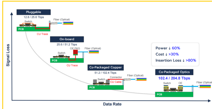
图表23：CPO 方案可降低 60% 的功耗和 30% 以上的成本
