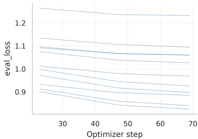
SimPO
