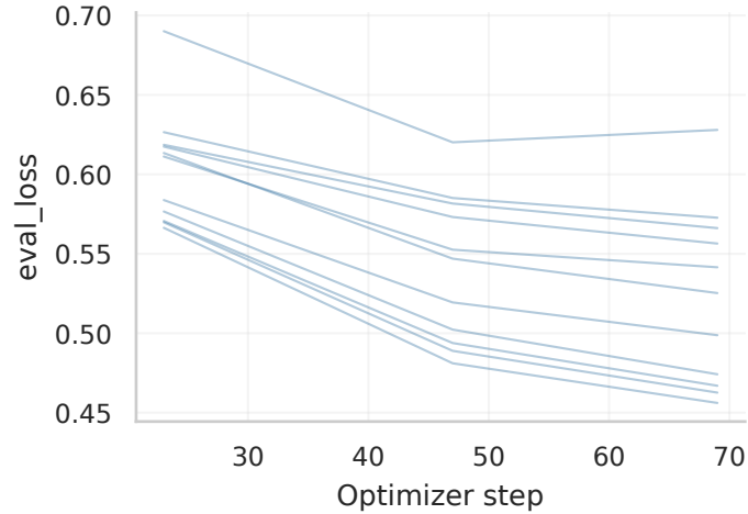
SimPO
