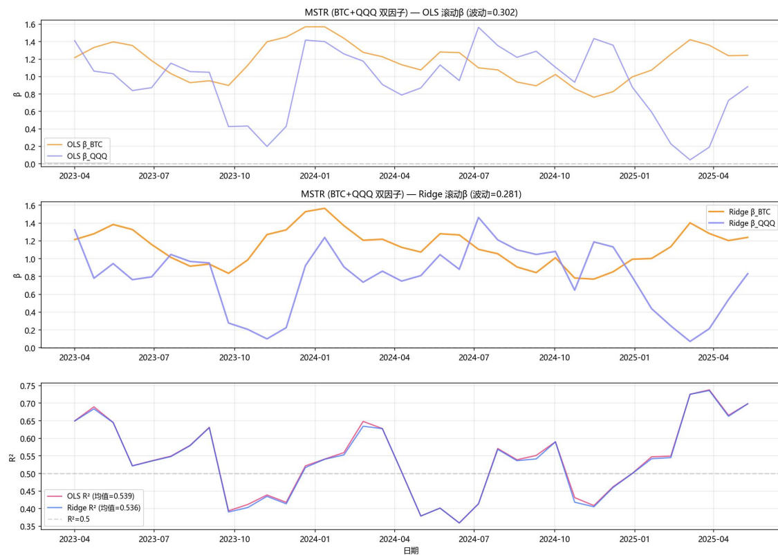
图 2-2: MSTR OLS vs Ridge Beta 对比
