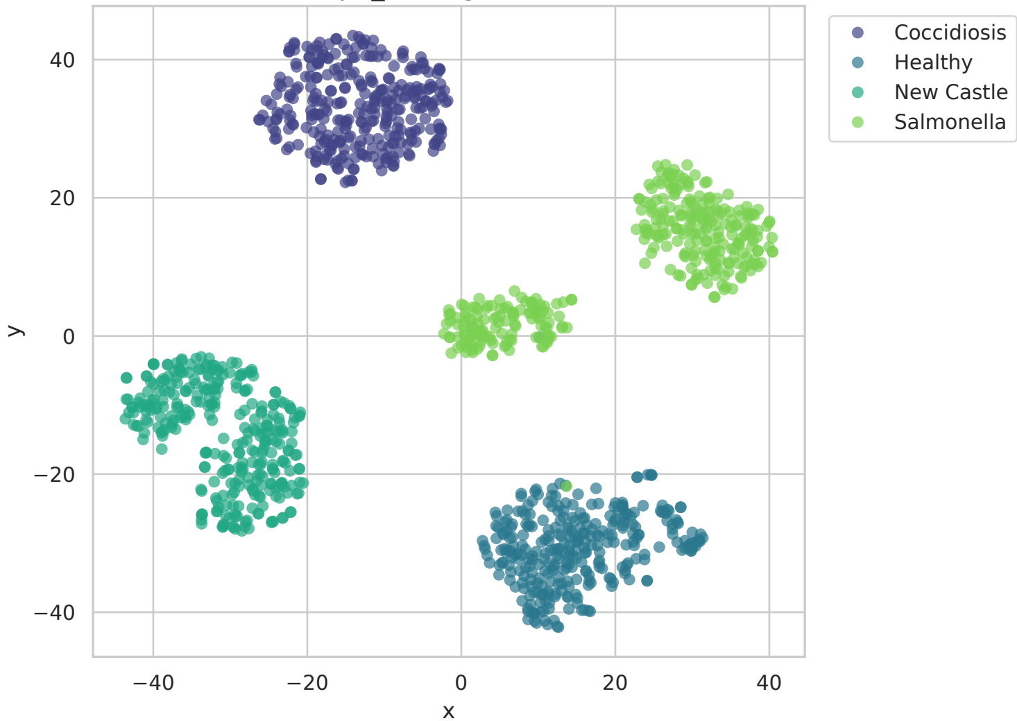
Exp1_Leakage - t-SNE
