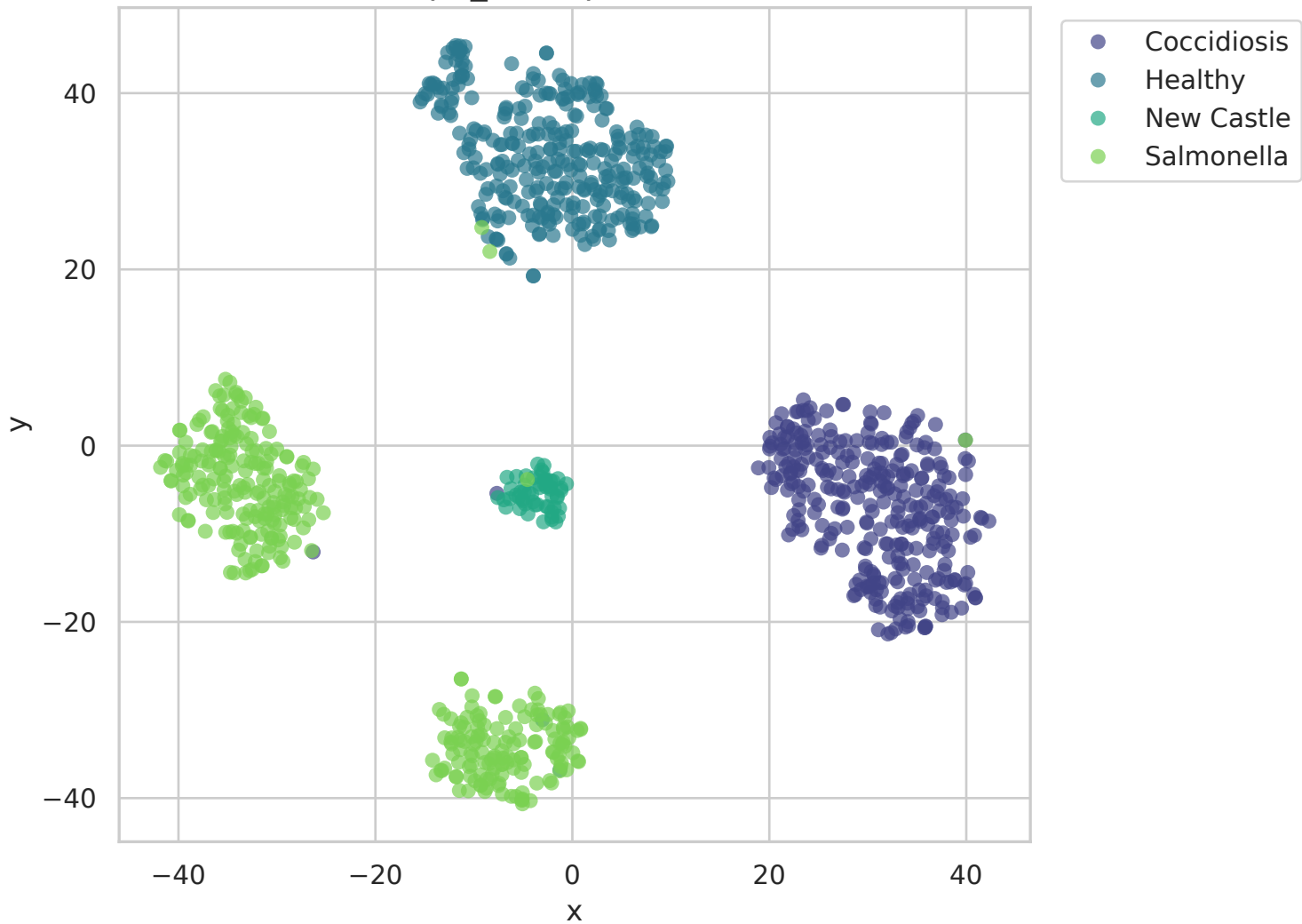
Exp2_CamSplit - t-SNE
