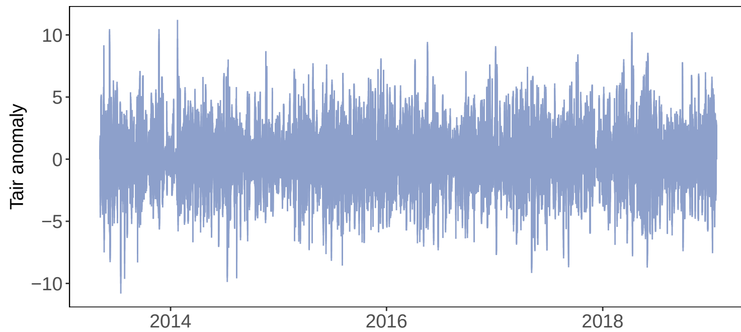
Tair anomaly
