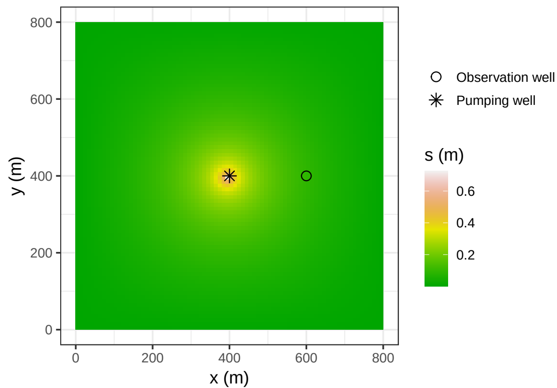
(d) 2D drawdown field t = 1000 s
