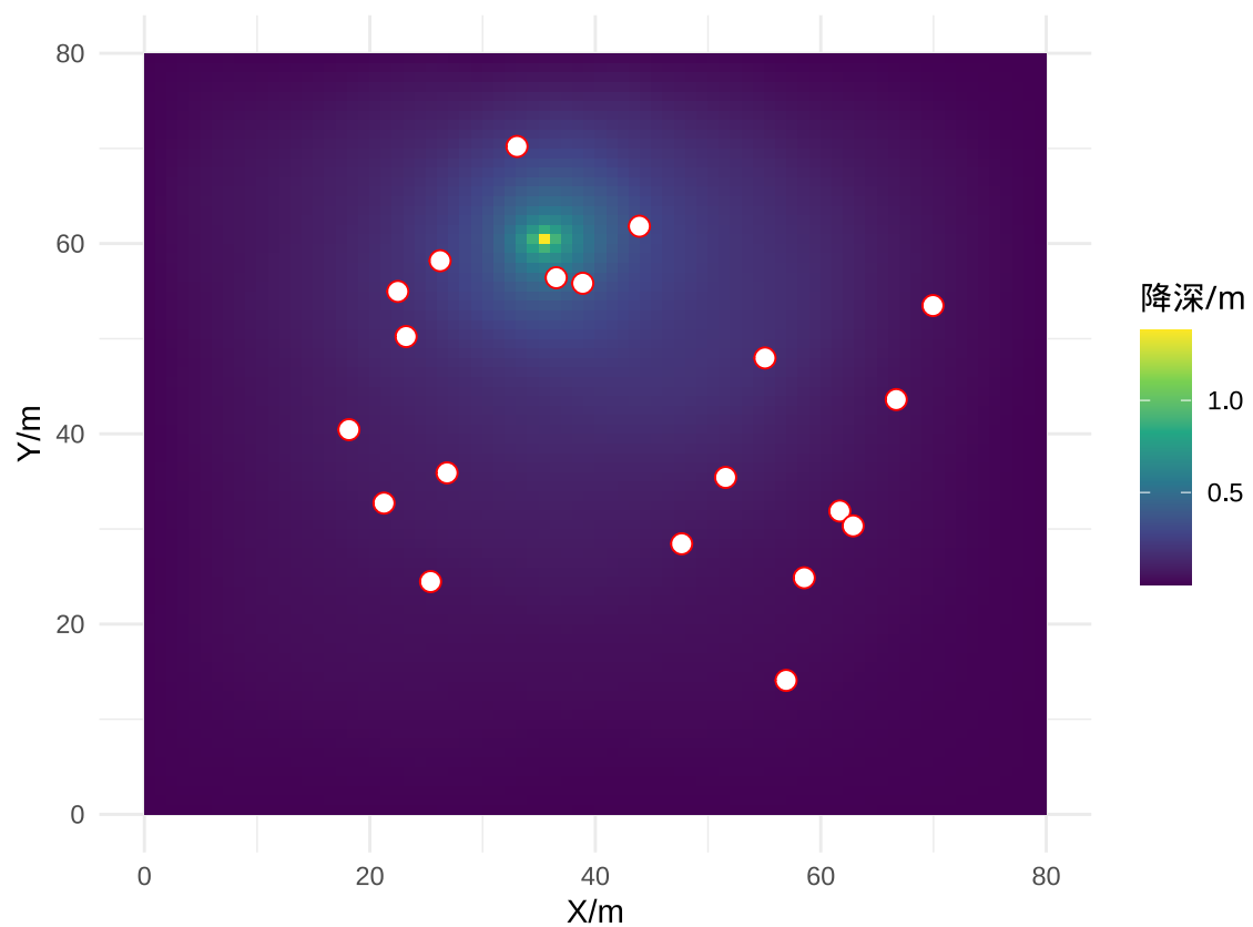
(b) 模拟降深及观测井
