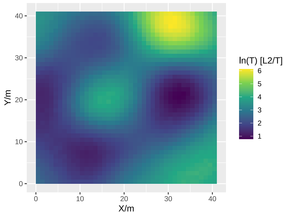
(d) 4次抽水试验
