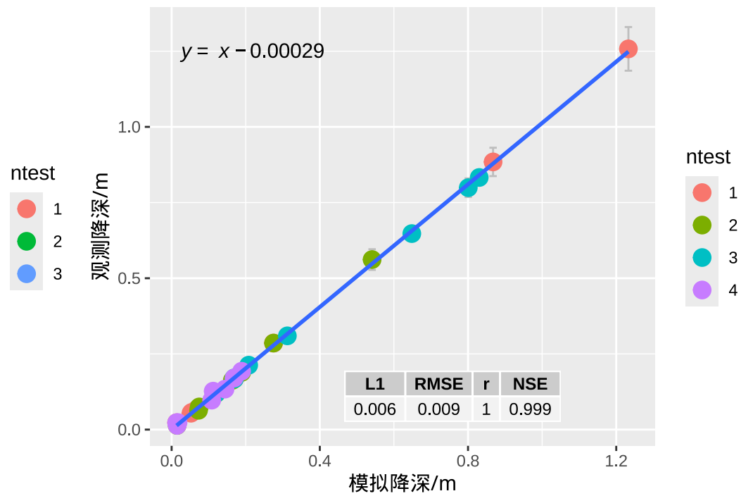
(d) 4次抽水试验
