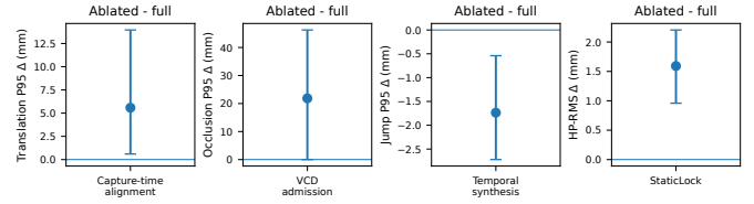
Figure 3: 组件消融的事件级配对差值（中位数与 IQR）。各面板使用独立纵轴；时序合成的 P95 为负，但其 P99 差值为正。
