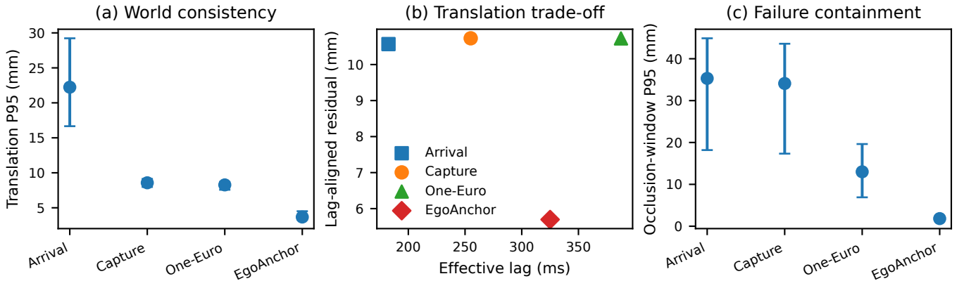
Figure 2: 实验一的核心行为表征。左：静止物体在主动头动下的平移 event-P95，反映世界一致性；中：持续平移中的有效时延与 lag-aligned residual，越靠左下越好；右：遮挡窗平移 P95，反映坏观测对已有锚点的破坏程度。误差棒表示事件级 IQR。
