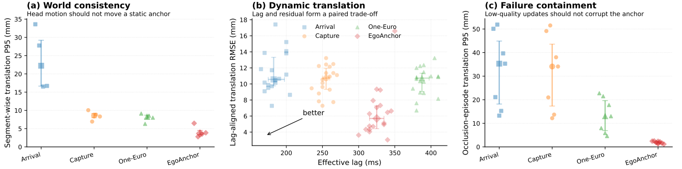
Figure 2: 实验一的核心系统行为。小标记表示重复动作片段或遮挡过程，大标记与误差棒表示 median-IQR。左：主动头动下的静止物体世界一致性；中：持续平移的 fitted-lag-aligned-residual 联合权衡，越靠左下越好；右：遮挡期间坏观测对已有锚点的破坏程度。左、右面板从零开始；权衡图按数据范围缩放。
