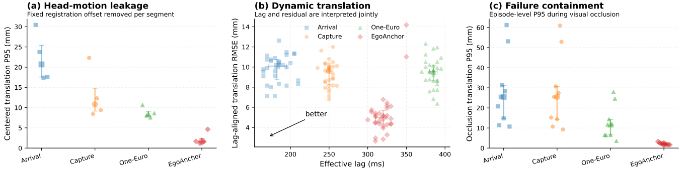
Figure 2: 新数据上的三项核心分布性结果。小标记表示重复动作片段或遮挡过程，大标记与误差棒表示 median-IQR。左：在每个片段内移除固定注册偏置后的头动泄漏；中：持续平移的 fitted-lag-aligned-residual 联合权衡，越靠左下越好；右：遮挡期间的 episode-level P95。静止帧间抖动、旋转护栏、灾难性失效率与起停转换代价在表 1 中完整报告。
