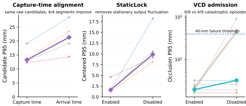
Figure 3: 目标化组件归因。左侧依次直接隔离采集时刻复合、StaticLock 与 VCD：采集时刻对齐比较同一原始候选的两种世界复合；StaticLock 比较中心化静止波动；VCD 面板使用对数坐标并标出 40 mm 灾难性阈值。右侧显示时序合成的 fitted-lag-aligned-residual 权衡。
