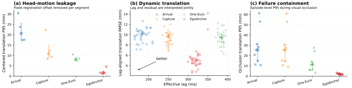
Figure 2: 新数据上的三项核心分布性结果。小标记表示重复动作片段或遮挡过程, 大标记与误差棒表示 median-IQR。左: 在每个片段内移除固定注册偏置后的头动泄漏; 中: 持续平移的 fitted-lag-aligned-residual 联合权衡, 越靠左下越好; 右: 遮挡期间的 episode-level P95。静止帧间抖动、旋转护栏、灾难性失效与起停转换代价在表 1 中完整报告。
