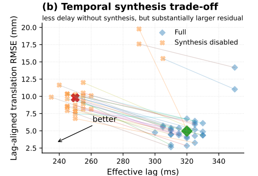
Figure 3: 目标化组件归因。左侧依次直接隔离采集时刻复合、StaticLock 与 VCD: 采集时刻对齐比较同一原始候选的两种世界复合; StaticLock 比较中心化静止波动; VCD 面板使用对数坐标并标出 40 mm 灾难性阈值。右侧显示时序合成的 fitted-lag-aligned-residual 权衡。
