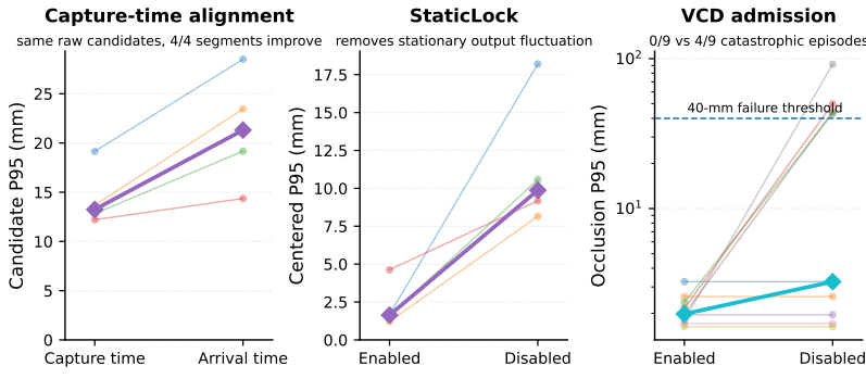
Figure 3: 目标化组件归因。左侧依次直接隔离采集时刻复合、StaticLock 与 VCD: 采集时刻对齐比较同一原始候选的两种世界复合; StaticLock 比较中心化静止波动; VCD 面板使用对数坐标并标出 40 mm 灾难性阈值。右侧显示时序合成的 fitted-lag-aligned-residual 权衡。
