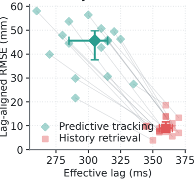
(d) Predictive tracking vs. history retrieval
