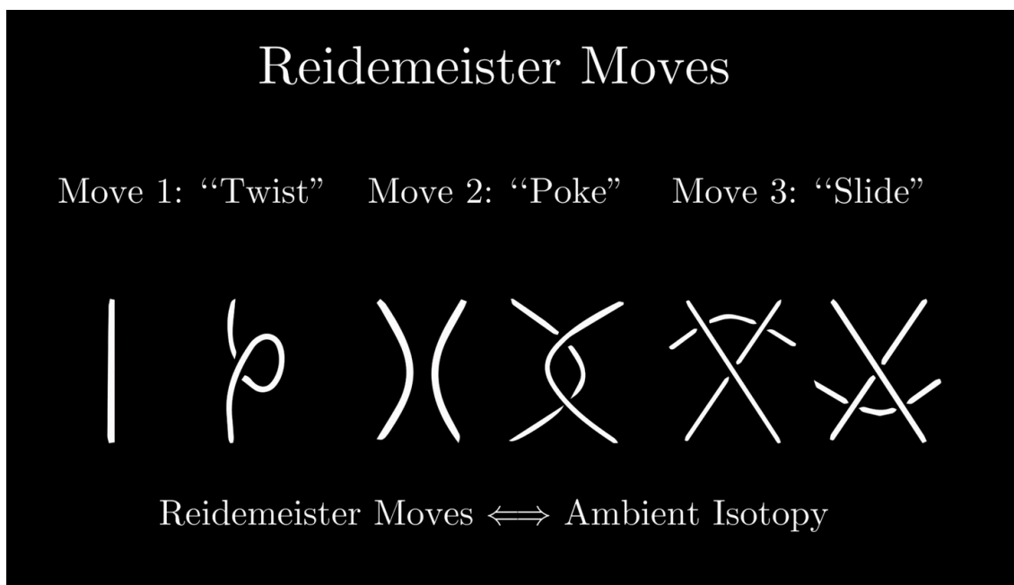
图 7. Reidemeister 运动
