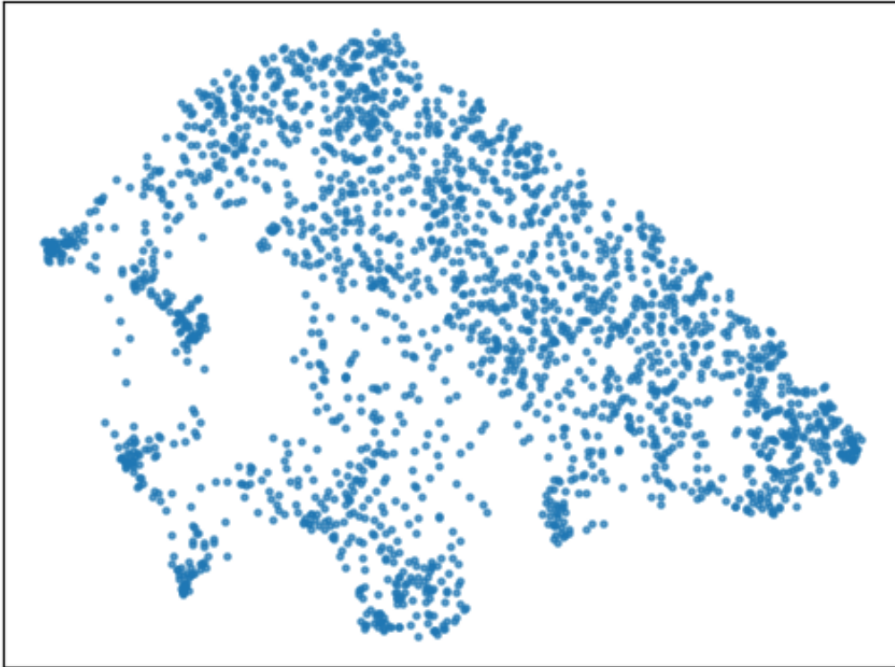
RaphaelMourad/Mistral-DNA-v1-422M-hg38
