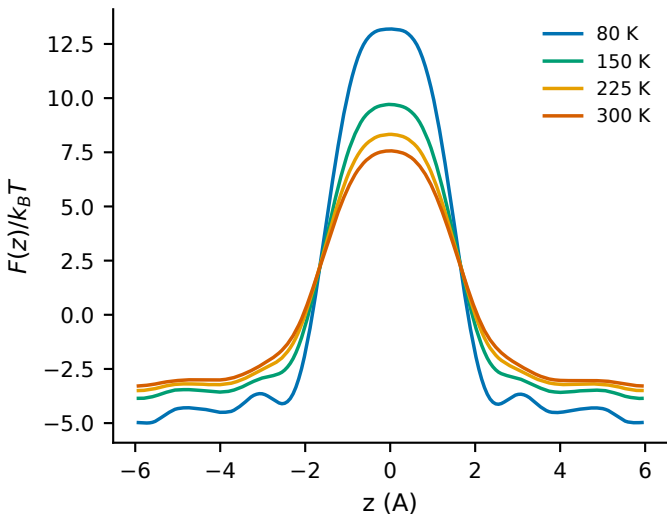
reference free energy per T
