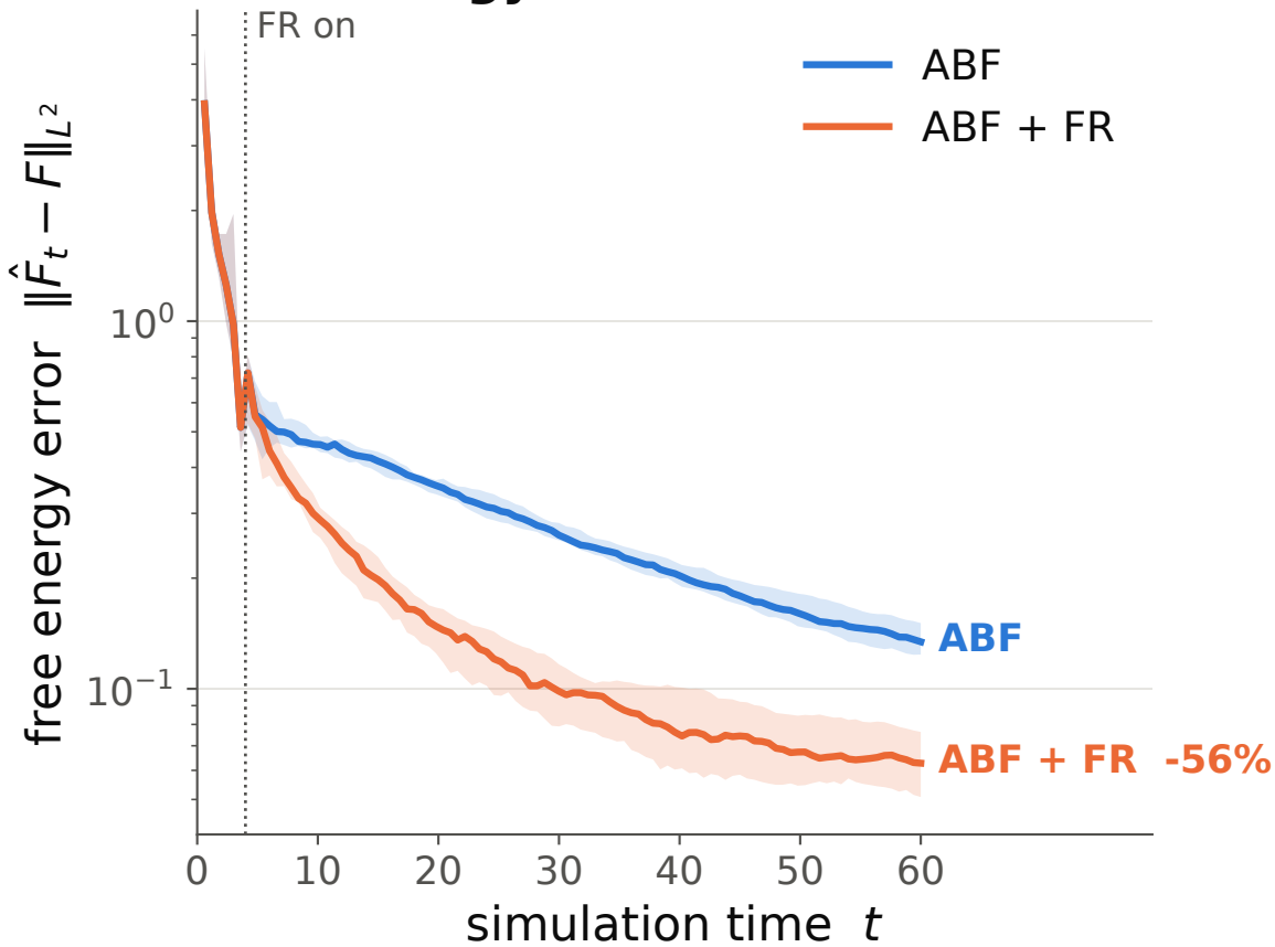
Free energy
