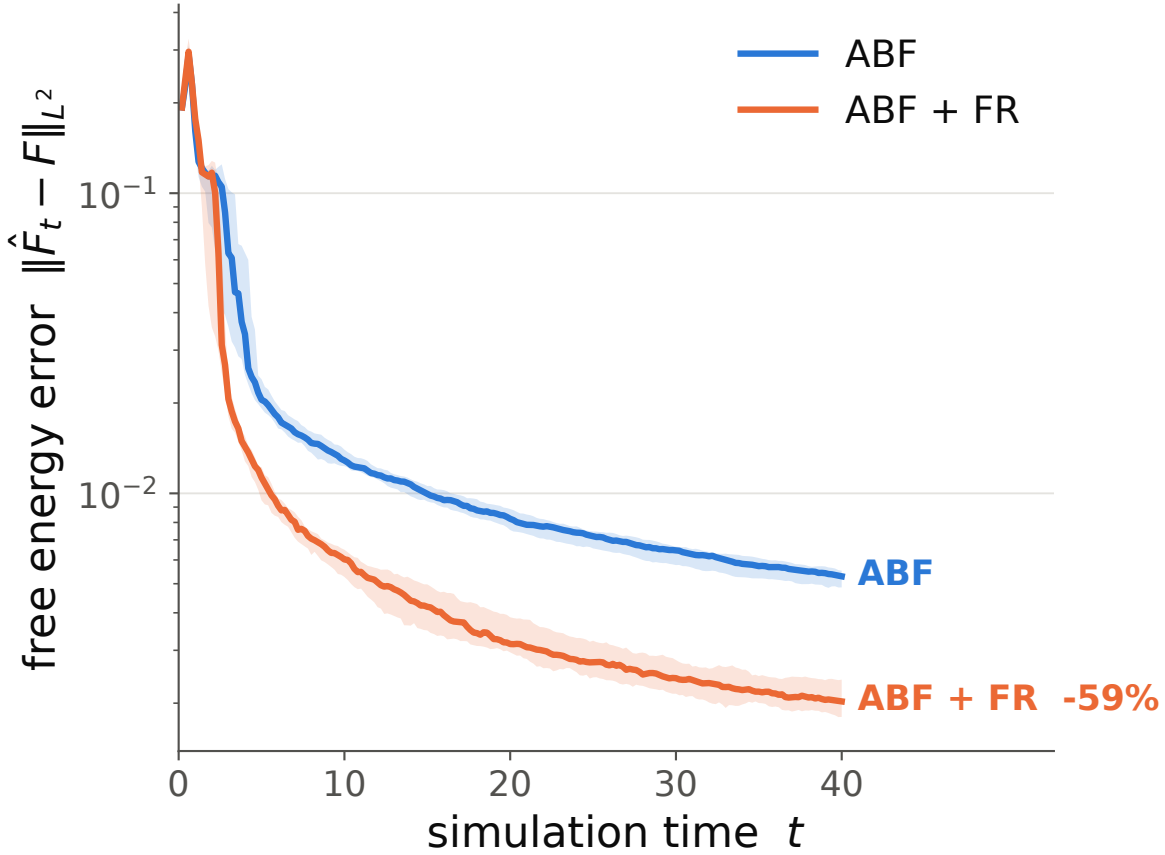
Free energy
