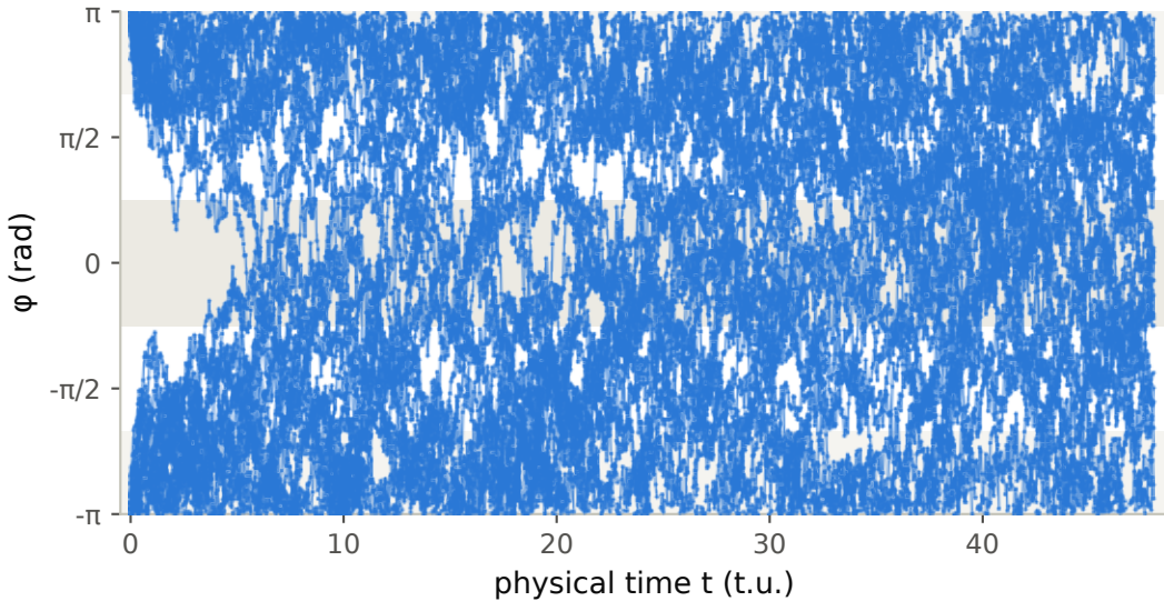
(c) ABF+FR · seed 30000 · slots 0-31 · first 48 t.u.
