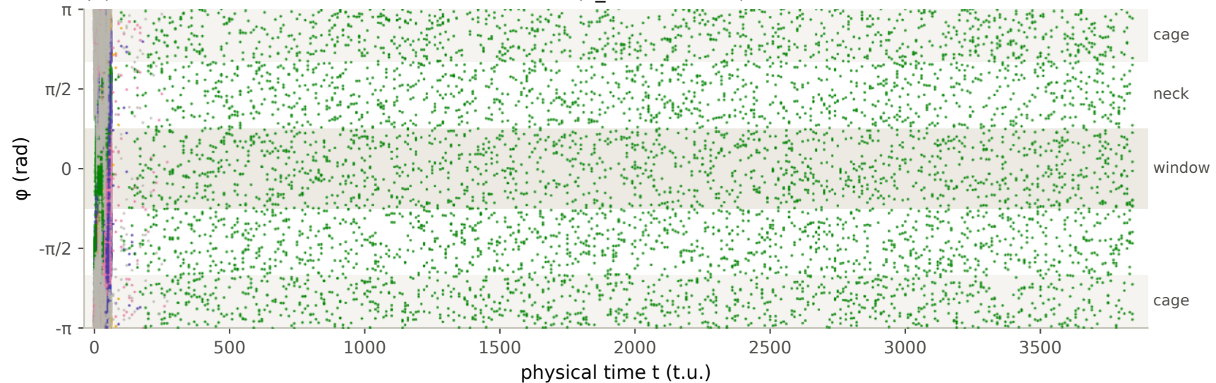
(d) ABF+FR · seed 15000 · slots 0-15 · whole run (T_N = 3840 t.u.)
