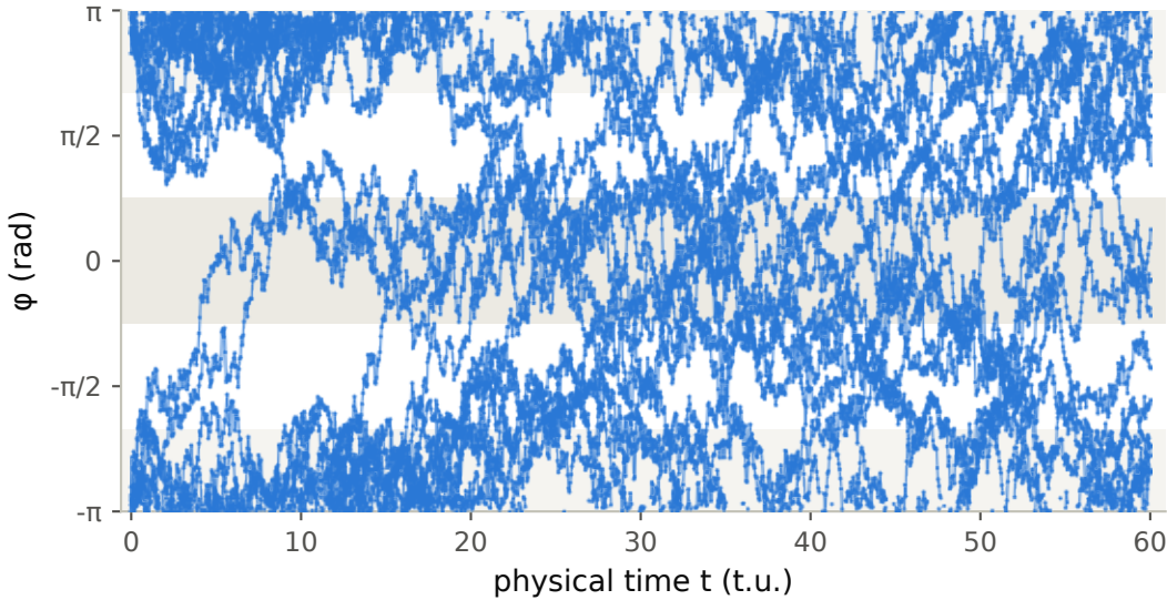
(c) ABF+FR · seed 15000 · slots 0-15 · first 60 t.u.
