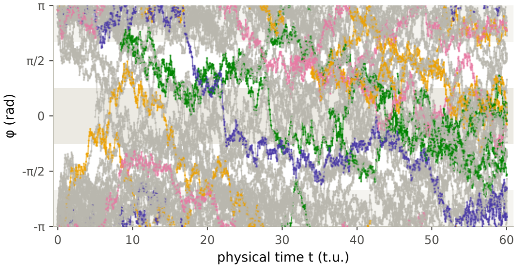
(c) ABF+FR · seed 15000 · slots 0-31 · first 60 t.u.
