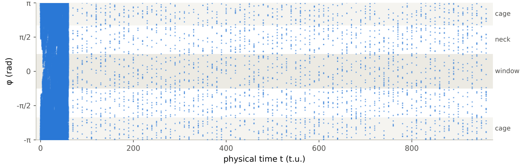
(d) ABF+FR · seed 15000 · slots 0-31 · whole run (T_N = 960 t.u.)
