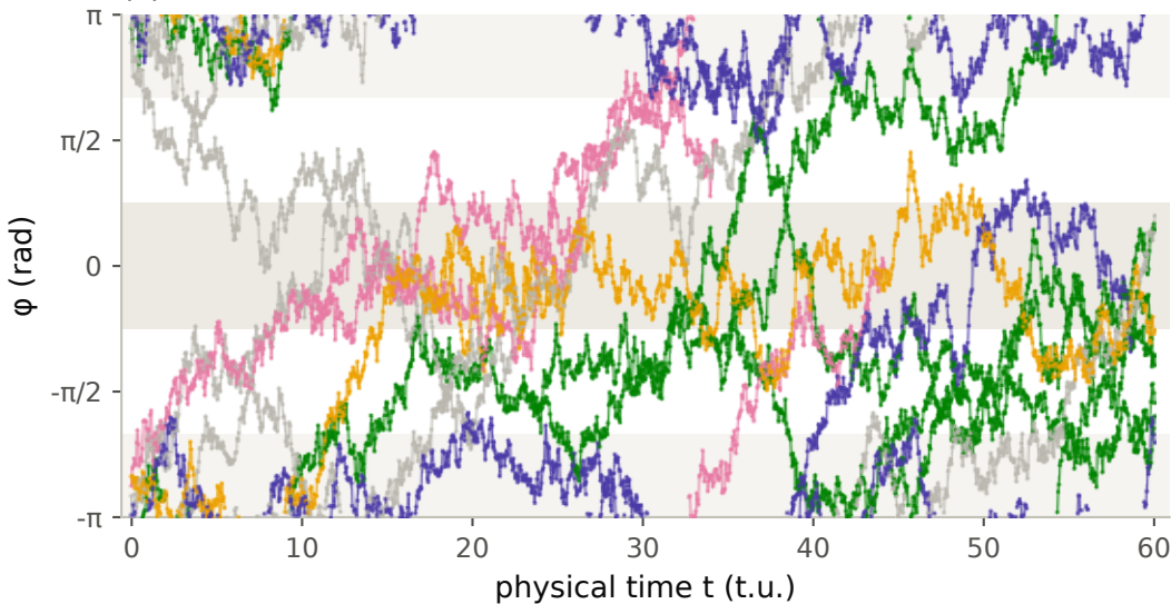
(c) ABF+FR · seed 15000 · slots 0-7 · first 60 t.u.
