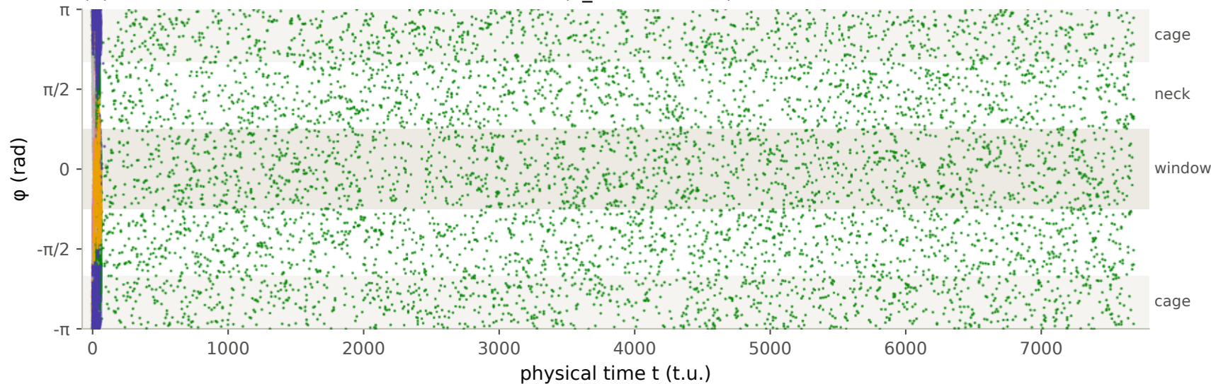
(d) ABF+FR · seed 15000 · slots 0-7 · whole run (T_N = 7680 t.u.)
