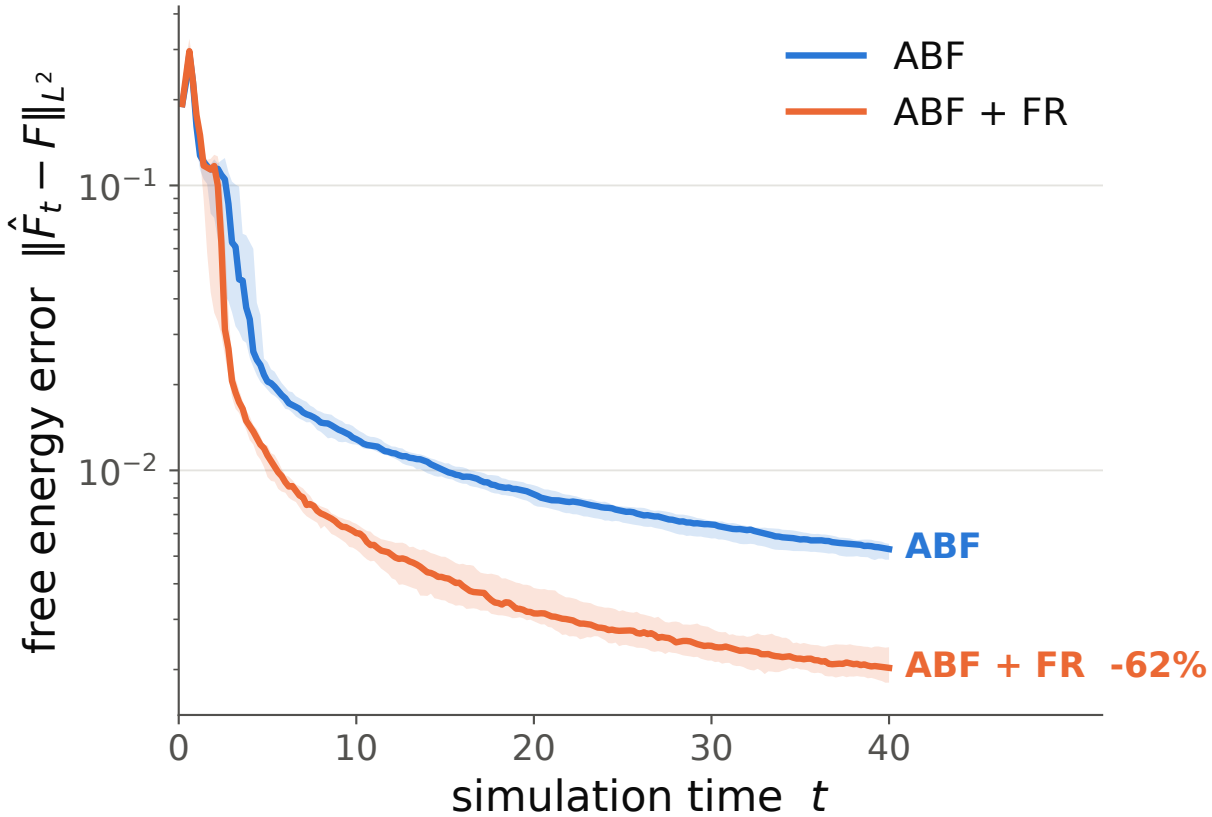
Free energy
