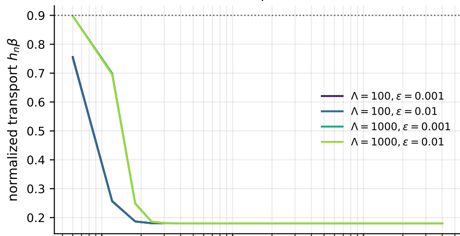
Gaussian posterior
