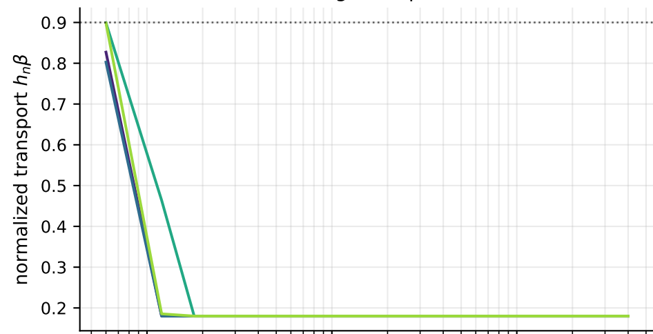
smooth log-cosh posterior
