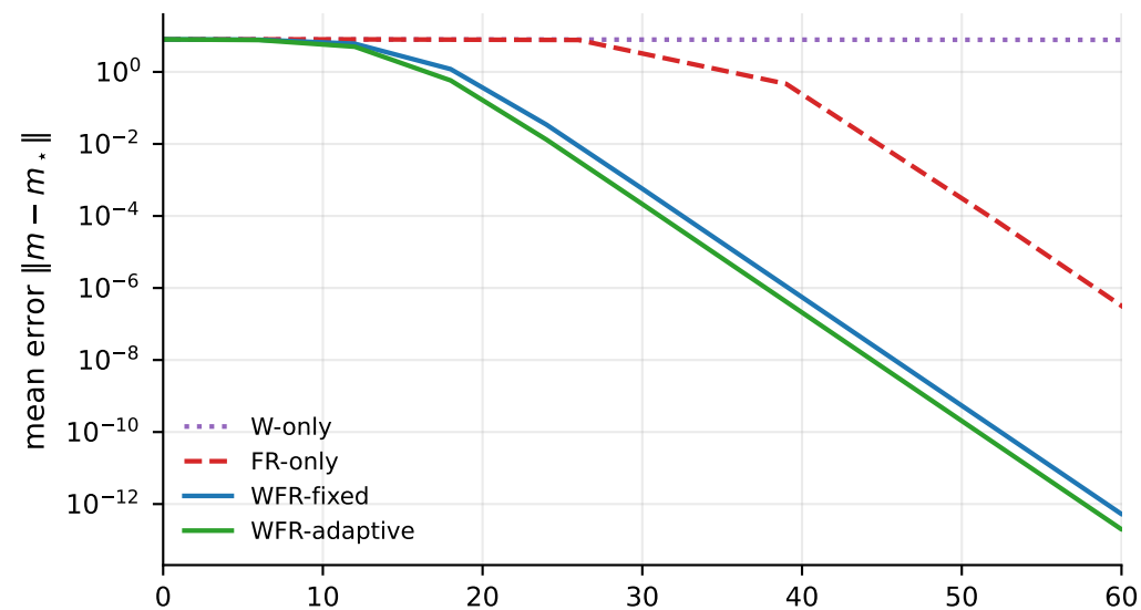
smooth log-cosh posterior ( \Lambda = 1000, \varepsilon = 10^{-3} )
