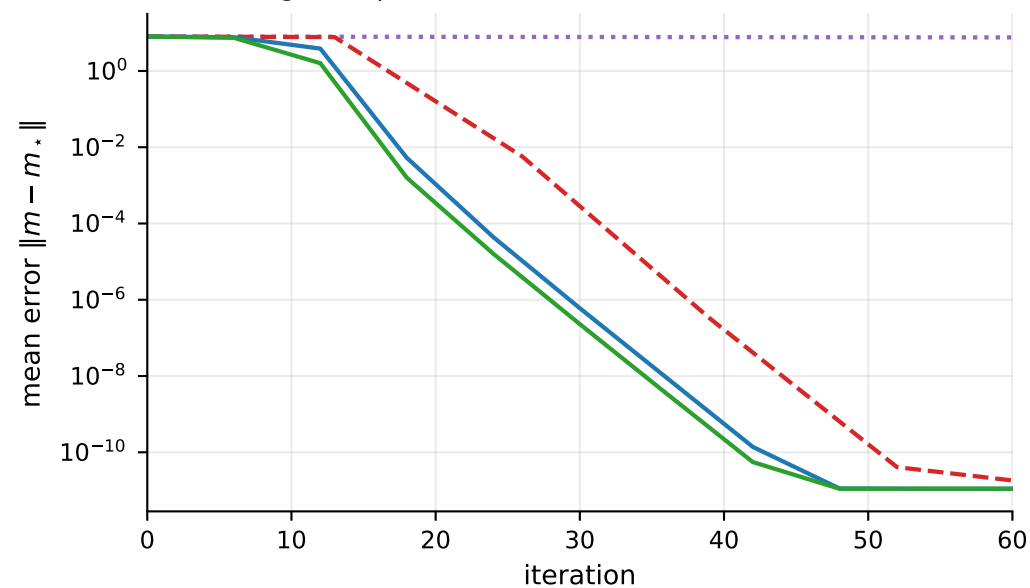
smooth log-cosh posterior ( \Lambda = 1000, \varepsilon = 10^{-3} )
