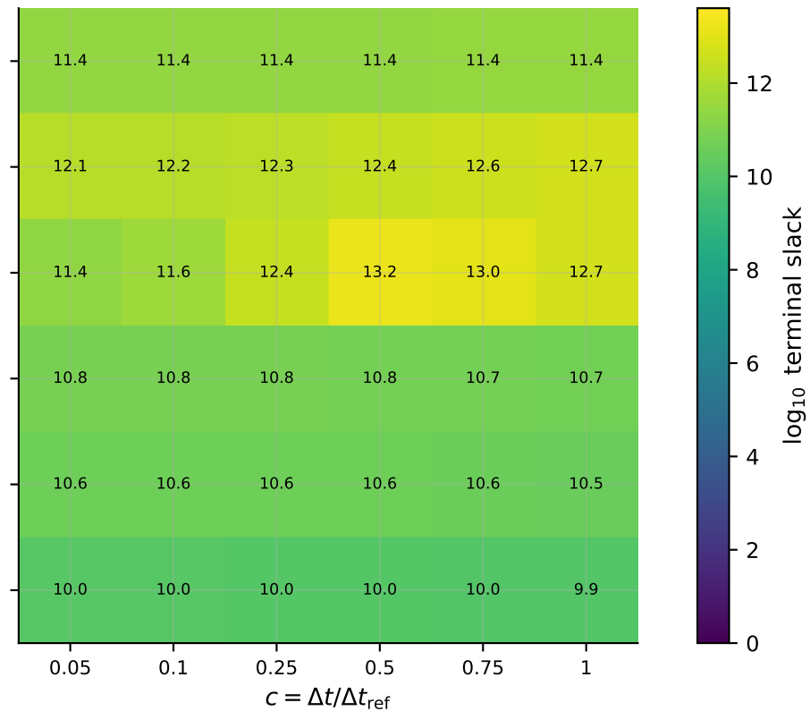
KL
