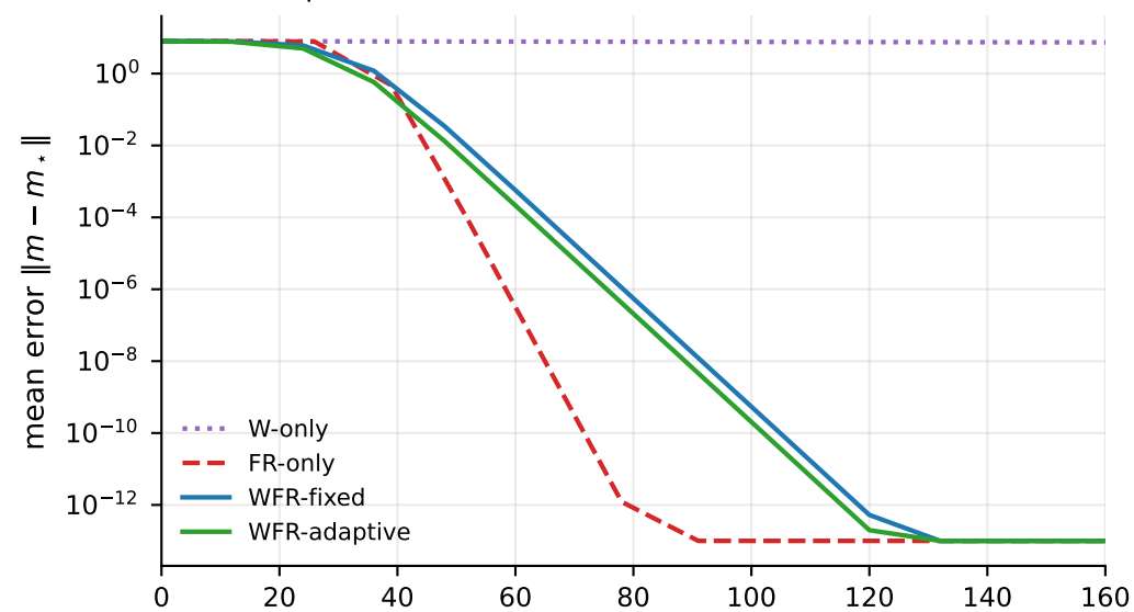
smooth log-cosh posterior ( \Lambda = 1000, \varepsilon = 10^{-3} )
