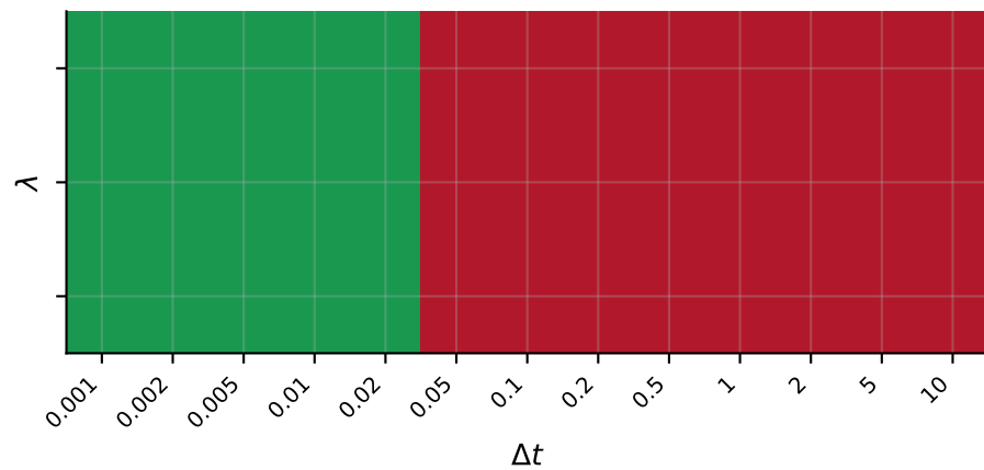
KL
