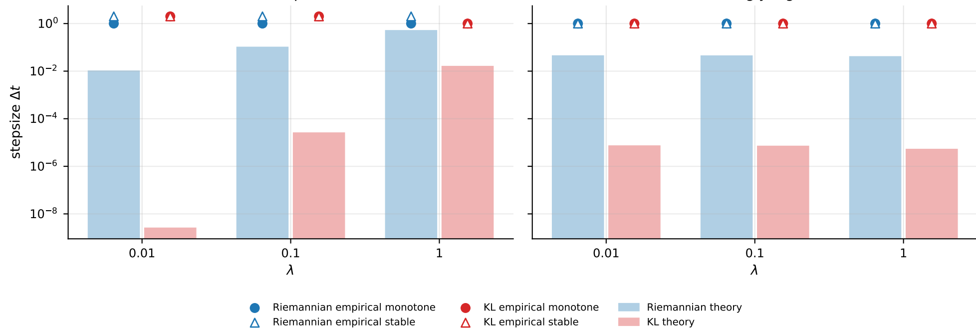
Gaussian posterior
