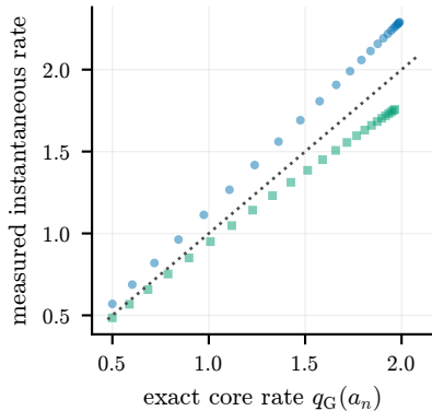
(b) Lemma 2.24 identity
