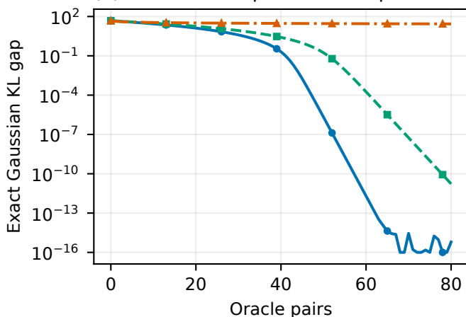
(d) Diao anisotropic Gaussian pilot
