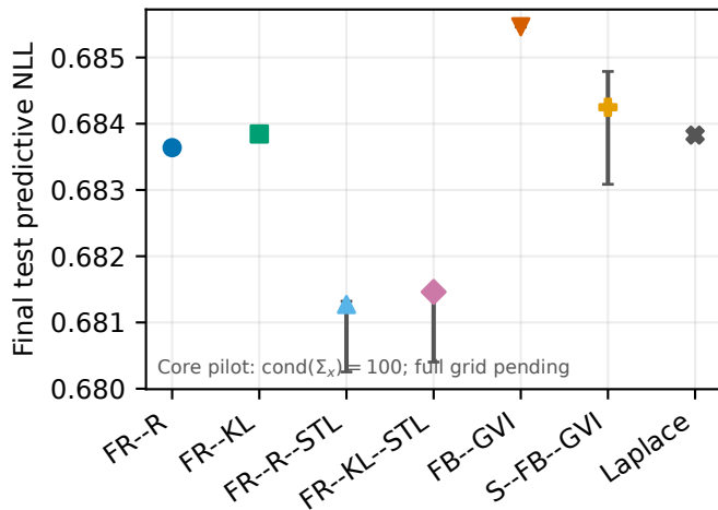
(d) Final NLL at condition 100
