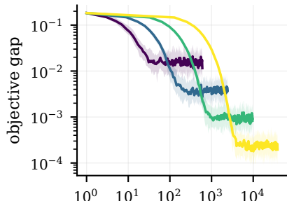
gradient-Hessian oracle pairs
