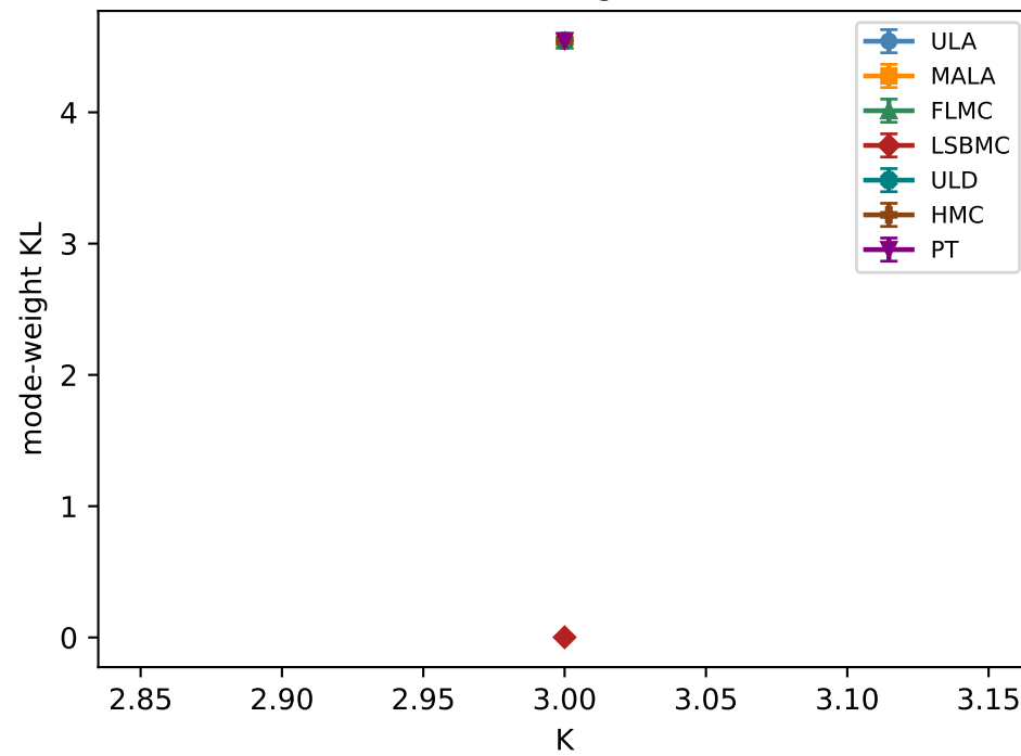
mode-weight KL
