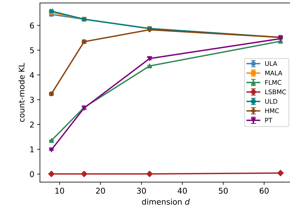
count-mode KL
