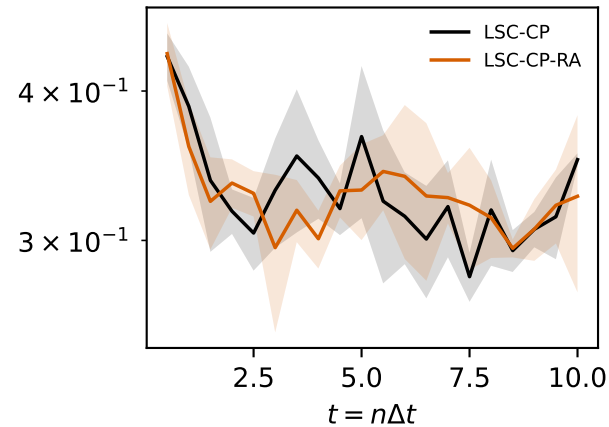
TV_density
