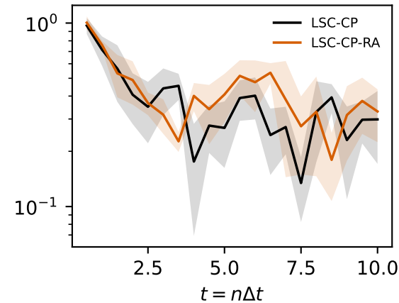
W2
