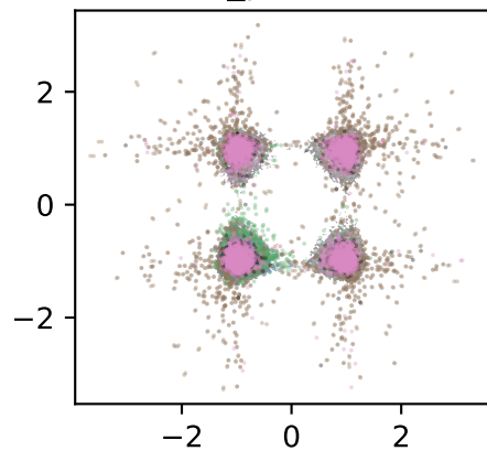
order_parameter
