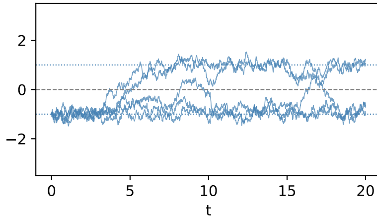
ULA
