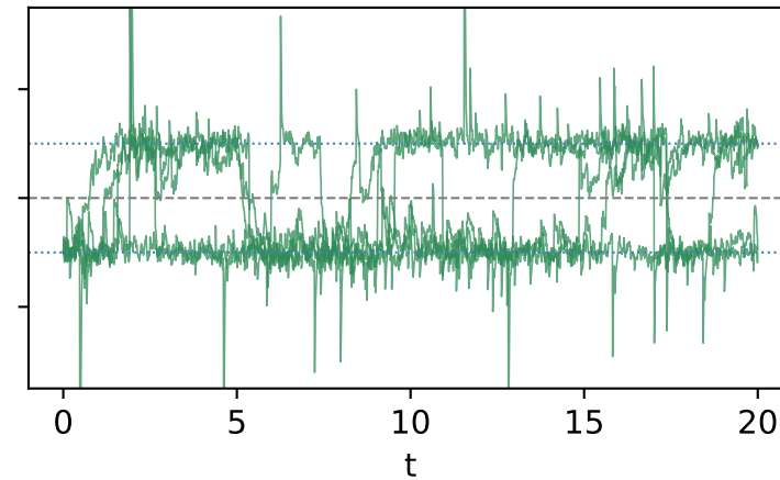
FLMC
