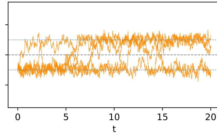
MALA
