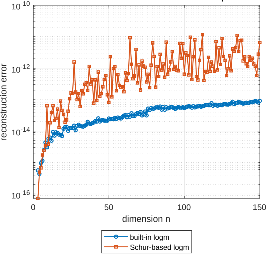
Reconstruction error: \|Q - \text{expm}(X)\|_F
