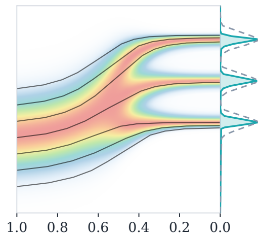
(b) TSR ( k=2, \sigma=1 )
