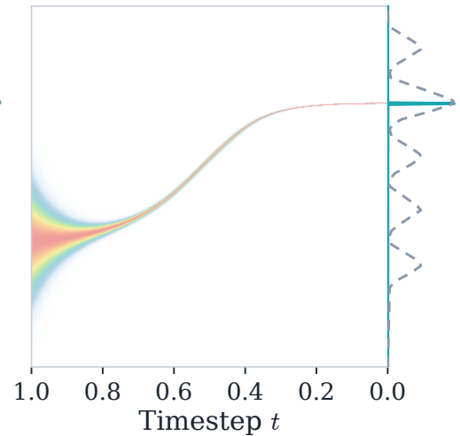
(d) TSR ( k=3 , \sigma \rightarrow \infty ) or \tau_{\text{score}} = 1/3
