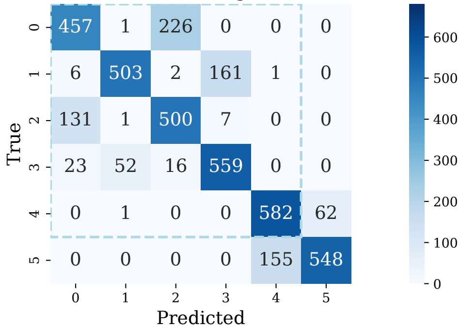
hierarchical-logiKNet
