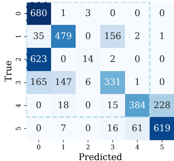
Vanilla-MLP
